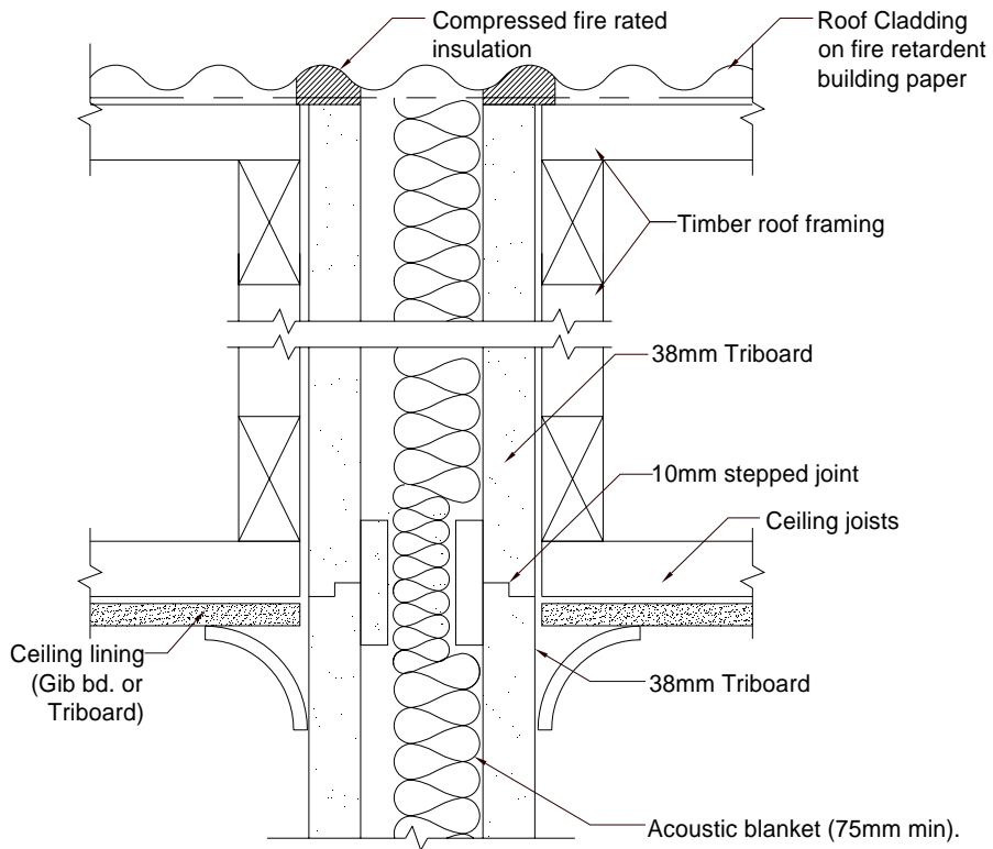
T i m b e r C e i l i n g
