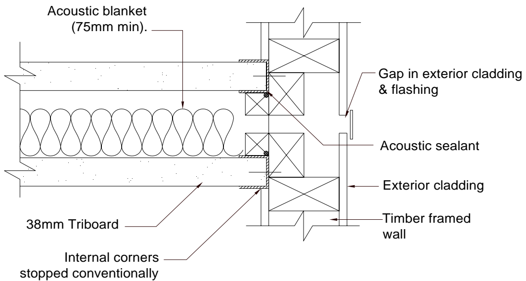
T i m b e r W a l l
